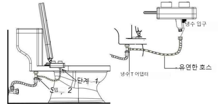
5. 냉수 공급 연결 비데에
