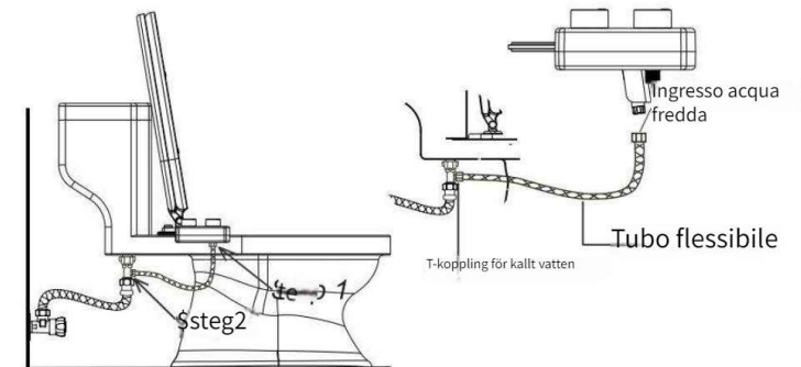
5. Anslut kallvattentillförseln bidet
