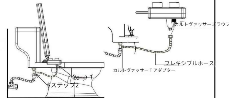
5. 冷水供給を接続する ツム ビデ
